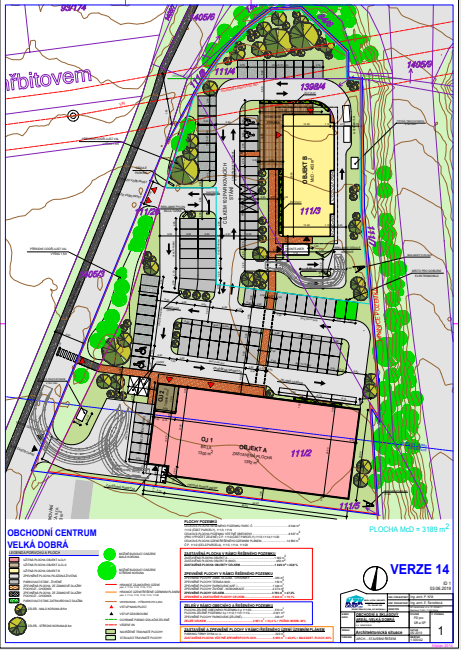
Architektonická studie plánovaného obchodního centra
